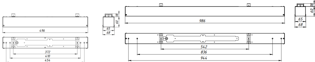
Рисунок 4 - Габаритные размеры при комплектации с креплением скоба 05908 светильников Trade Linear 490x65x60 (слева) и Trade Linear 980x65x60 (для моделей 1472мм и 1962мм установка креплений аналогичная).
